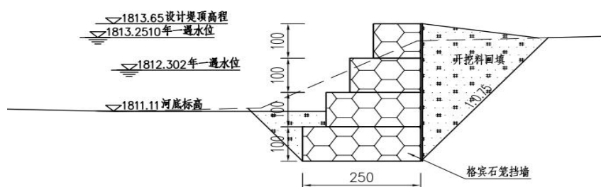
图2-6 格宾石笼挡墙断面图
