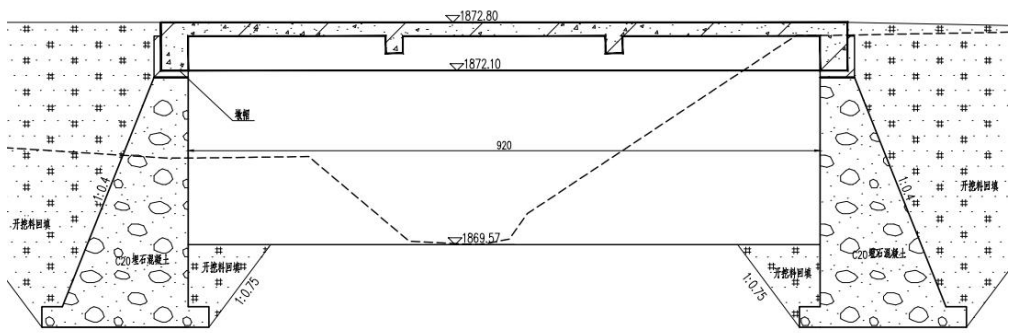
图2-7 机耕桥横断面示意图
