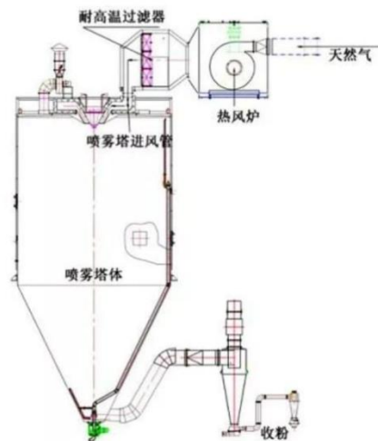
图 2-4 喷雾干燥塔主体结构布置图
