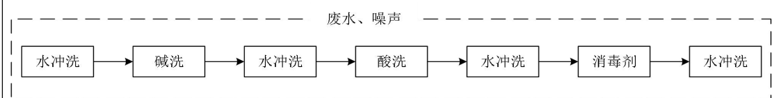
图 2-2 CIP 清洁工艺流程及产污节点图
