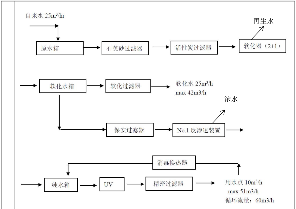
图 2-9 纯水制备工艺流程图
