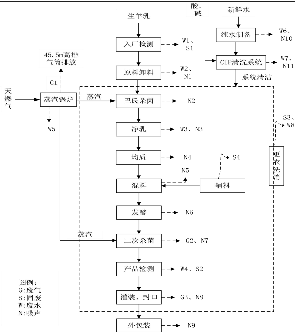
图 2-3 酸羊奶生产工艺流程及产污节点图
