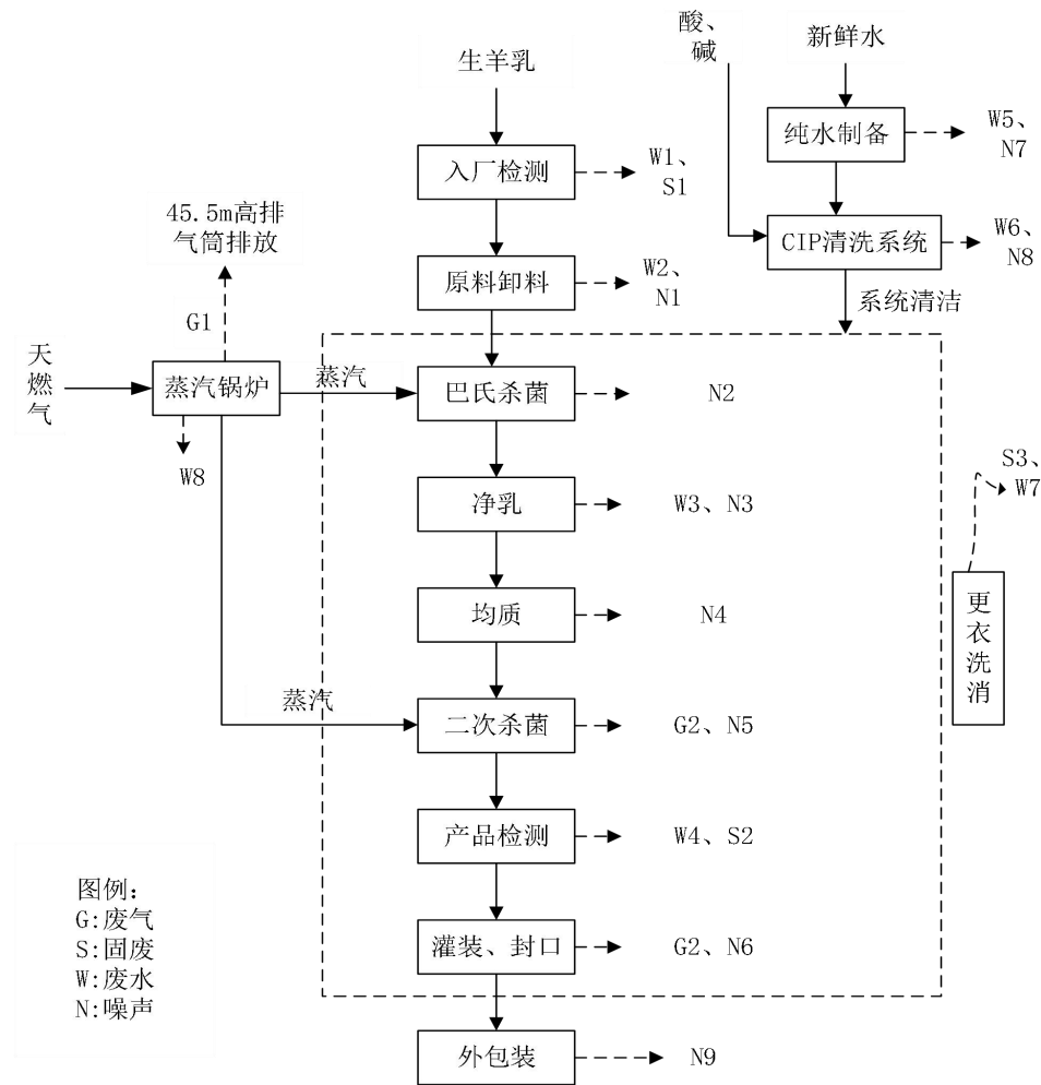
图 2-1 鲜羊乳生产工艺流程及产污节点图
