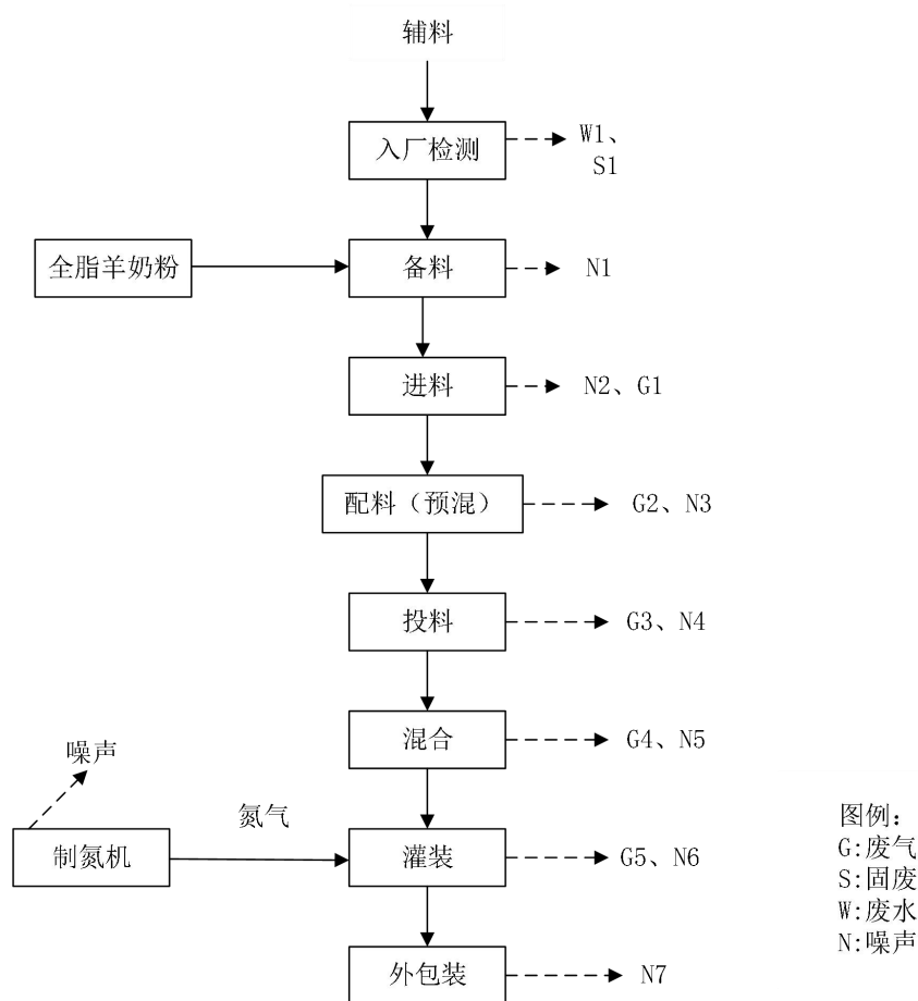
图 2-6 调制奶粉生产工艺流程及产污节点图
