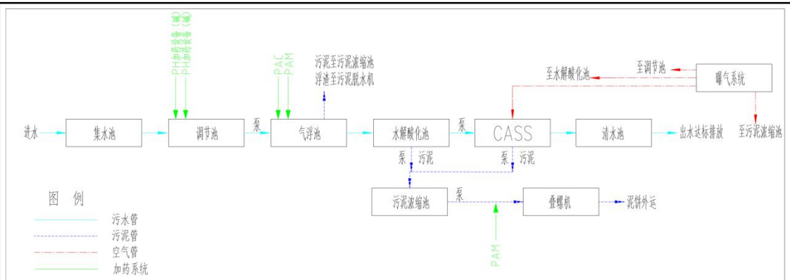
图 2-8 生产废水处理工艺流程图
