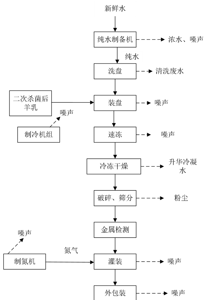
图 2-7 初乳粉生产工艺流程及产污节点图
