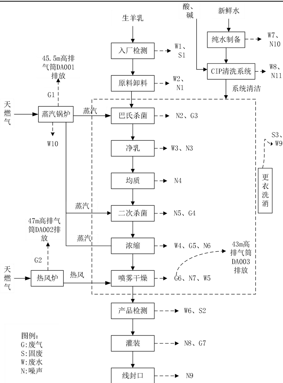
图 2-5 全脂羊奶粉生产工艺流程及产污节点图
