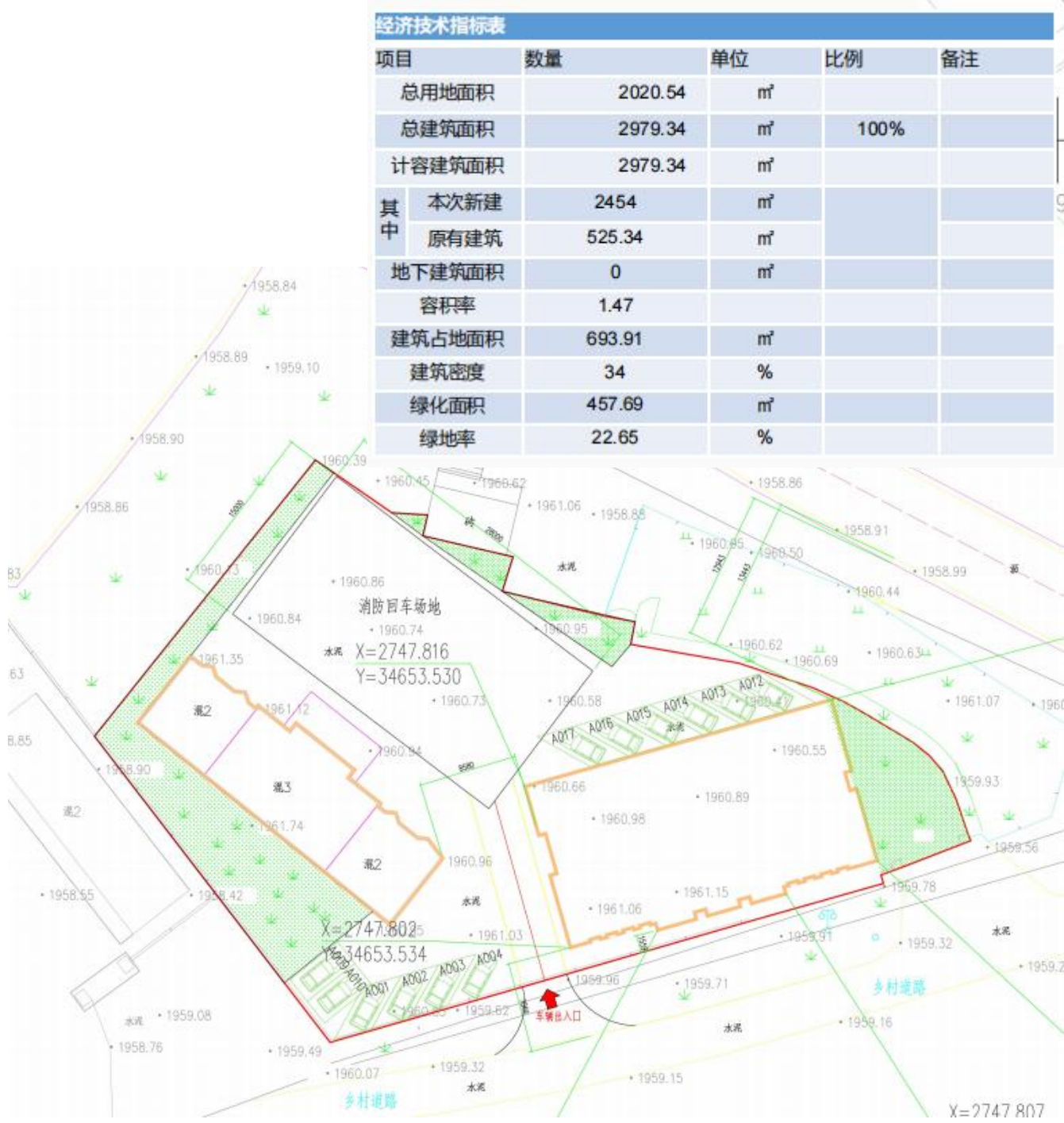
总平面图
