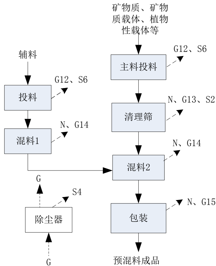
图 2-7 预混料生产线工艺流程及产污环节图
