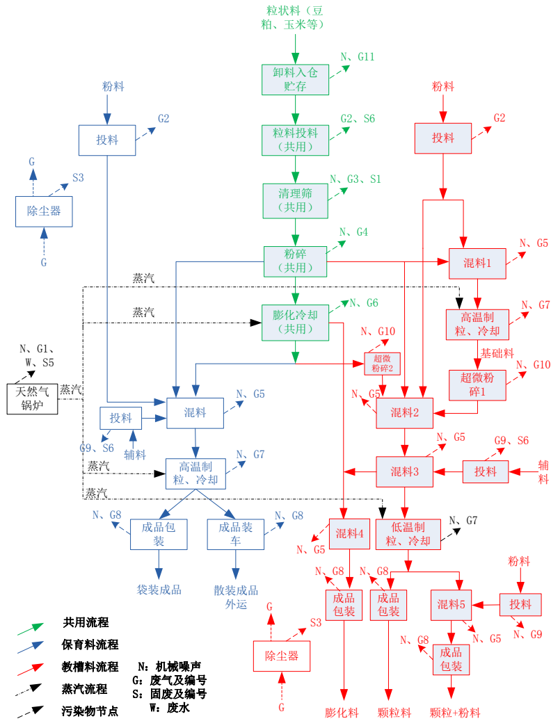
图 2-6 教槽料及保育料生产线工艺流程及产污环节图
