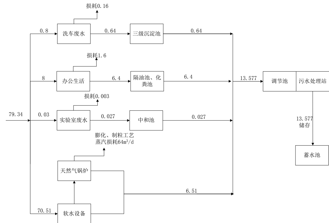
图 2-2 全厂雨天水量平衡图 单位 \text{m}^3/\text{d}
