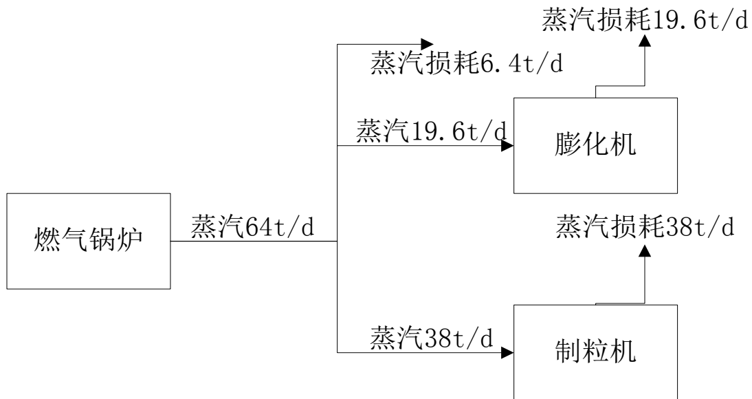
图 2-4 项目蒸汽平衡图
