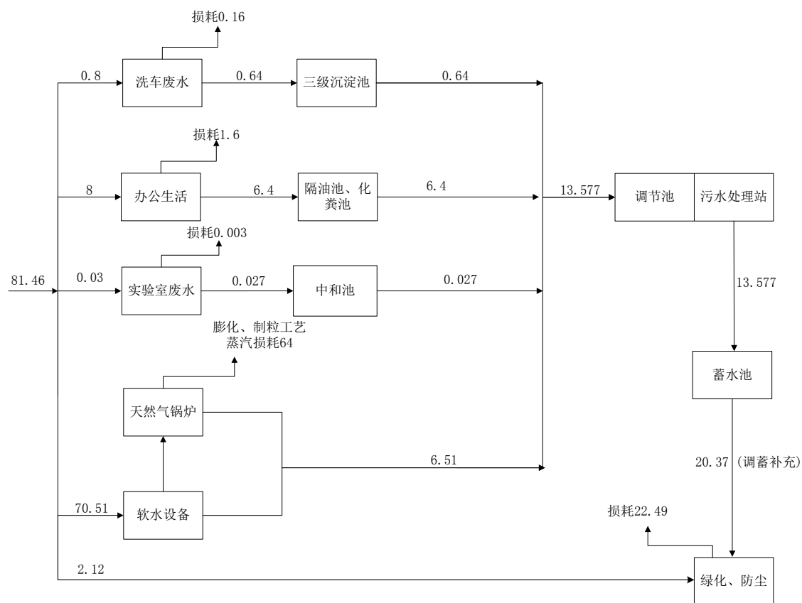
图 2-1 全厂非雨天水量平衡图 单位 \text{m}^3/\text{d}
